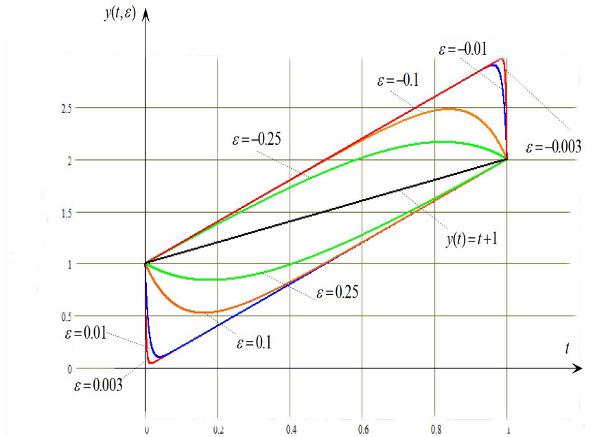
Рис. 1. Графики решений краевой задачи для различных \varepsilon .
